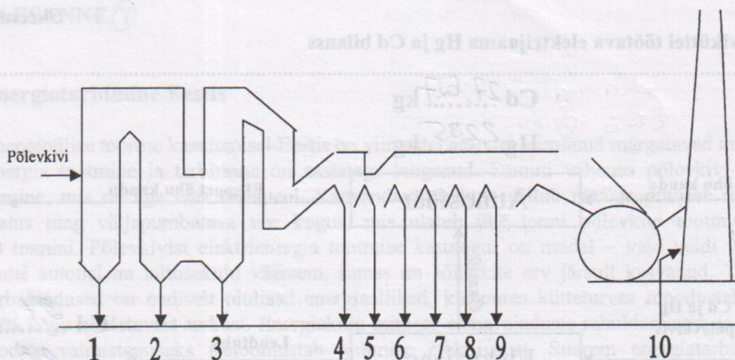
Joonis 1. Põlevkivikolde TP-101 ja selle suitsugaaside trakti skeem koos tuha proovivõtu kohtadega (Eesti Elektri jaam): 1 – koldetuhk, 2 – I gaasikäik (auru ülekuumendi), 3 – II gaasikäik (ökonomaizer), 4 – tsüklon, 5 – elektrifiltri eelkamber, 6–9 – elektrifilter, 10 – korstna lendtuhk
