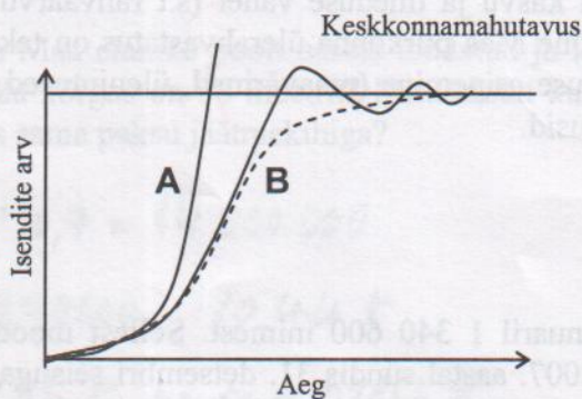
Joonis 1. Populatsiooni kasvu iseloomustavad kõverad. Pidevjoon B iseloomustab populatsiooni, mis ületab keskkonnamahutavuse ning isendite arvukus väheneb järsult, lisandub siis taas jne, kuni jääb püsima keskkonnamahutavuse tasemele. (Ökoloogialeksikon, 1992, lk 198)
